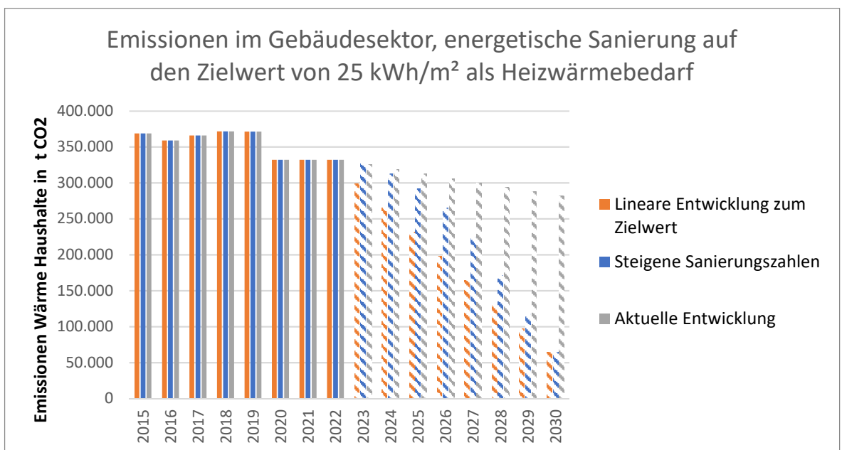
Abbildung 12: Szenarien zur Entwicklung der Emissionen im Gebäudesektor bei einem Standard von 25 kWh/m 2 als Heizwärmebedarf
