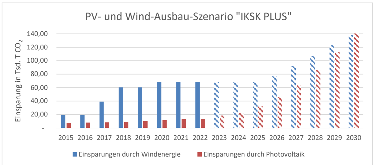
Abbildung 9: PV- und Wind-Ausbau-Szenario „IKSK PLUS“
