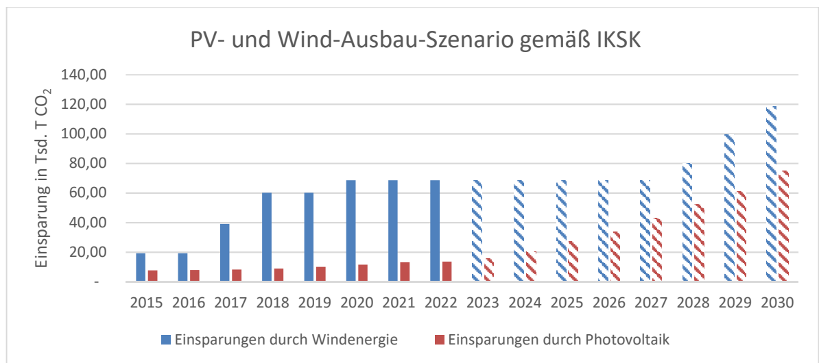
Abbildung 8: PV- und Wind-Ausbau-Szenario gemäß IKS, Quelle Daten 2015-2022: Marktstammdatenregister Bundesnetzagentur
