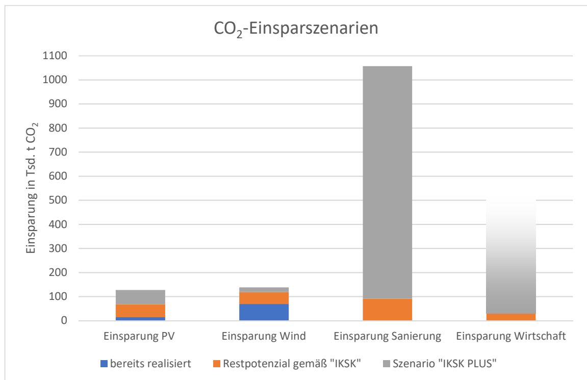
Abbildung 13: Zusammenfassung der Einsparszenarien im Sektor PV-Energie, Windenergie, Sanierung und Wirtschaft
