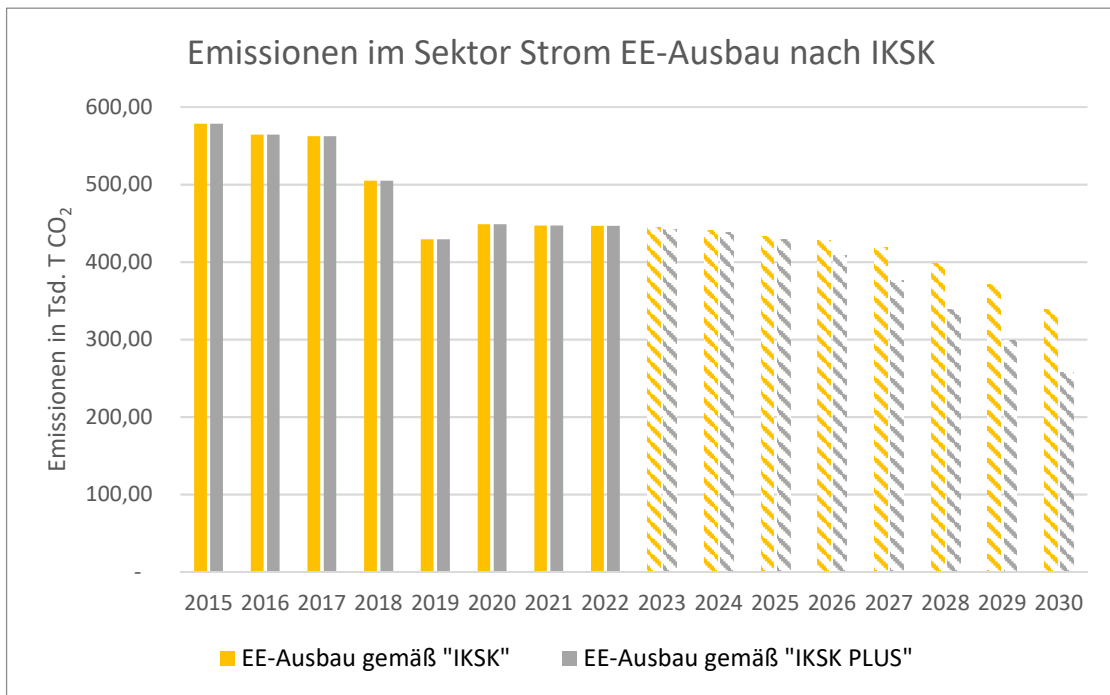
Abbildung 10: Emissionen und mögliche Entwicklungen im Bereich Strom bei EE-Ausbau nach Szenario „IKS“ und „IKS PLUS“, Quelle Daten 2015-2020: Energie- und CO 2 -Bilanz der Stadt Aachen 2020
